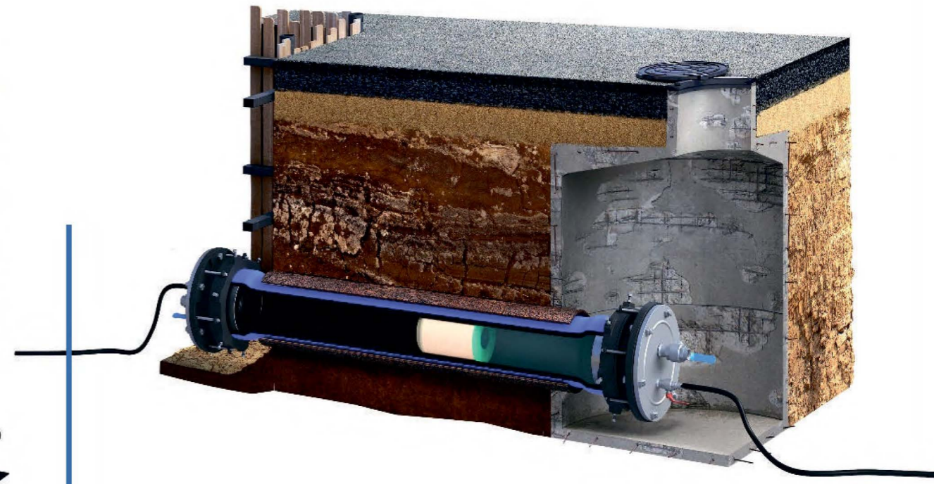
7 Реверсия ПЭ трубы
