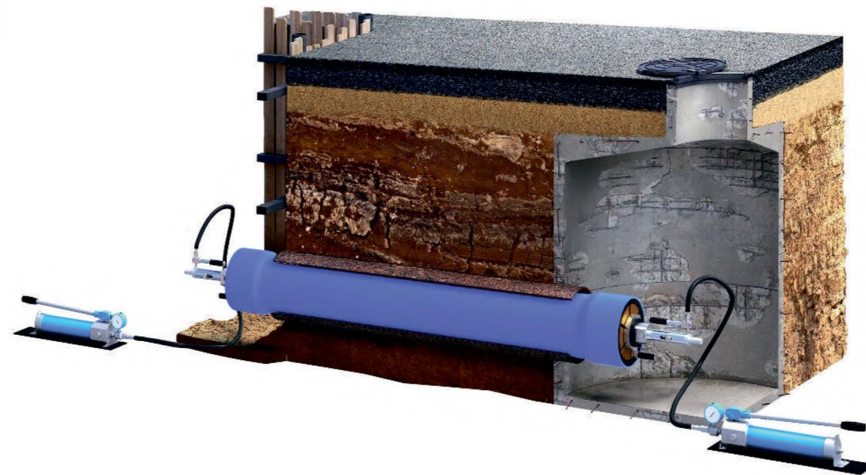
6 Реверсия ПЭ трубы
