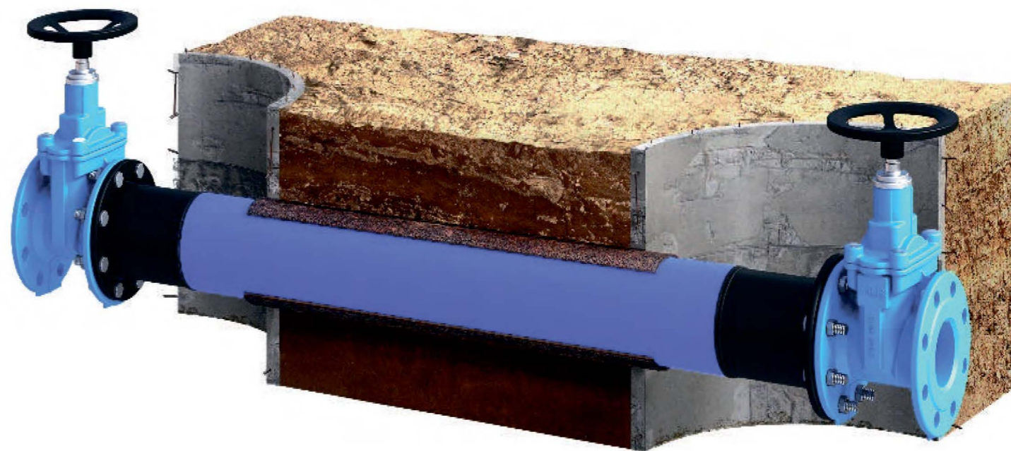
9 Монтаж запорной арматуры
